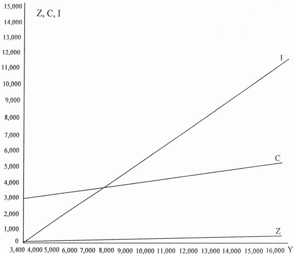
Rajah 3: Hubungan Antara Pendapatan (Y) Dengan Zakat (Z), Penggunaan (C), dan Pelaburan (I)
